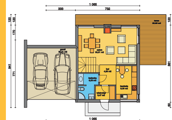
Rzut parteru – 86,00 m 2
