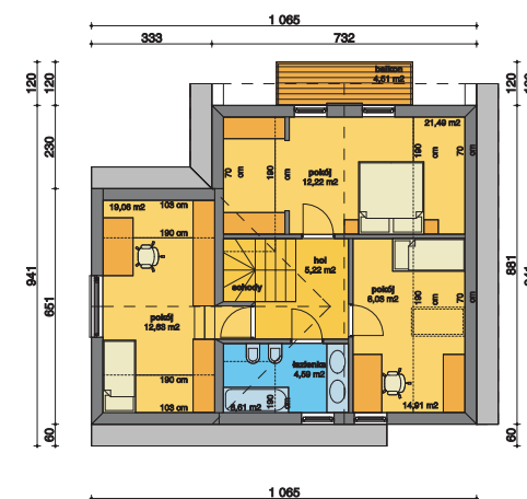
Rzut piętra – 42,70 m 2 (powierzchnia podłogi 67,30 m 2 )
