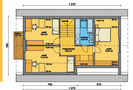
Rzut piętra – 49,70 m 2 (powierzchnia podłogi 70,60 m 2 )
