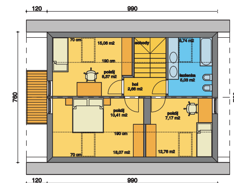
Rzut piętra – 33,60 m 2 (powierzchnia podłogi 57,30 m 2 )
