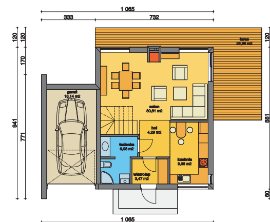
Rzut parteru – 71,30 m 2
