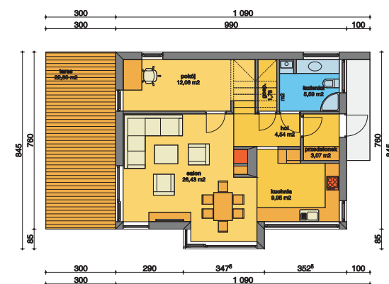
Rzut parteru – 63,40 m 2
